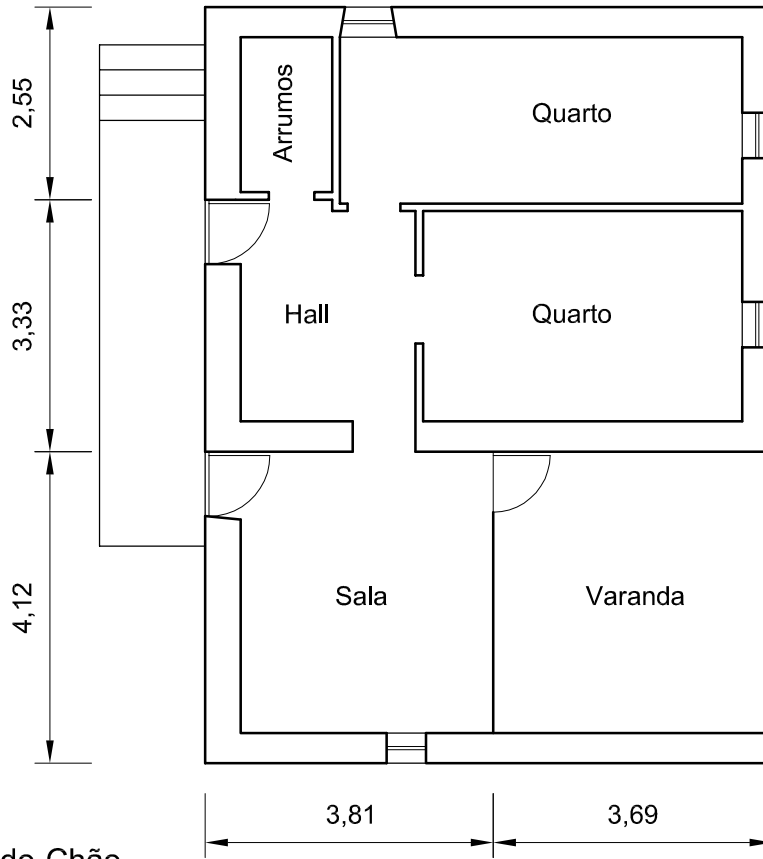
Planta do Rés-do-Chão
